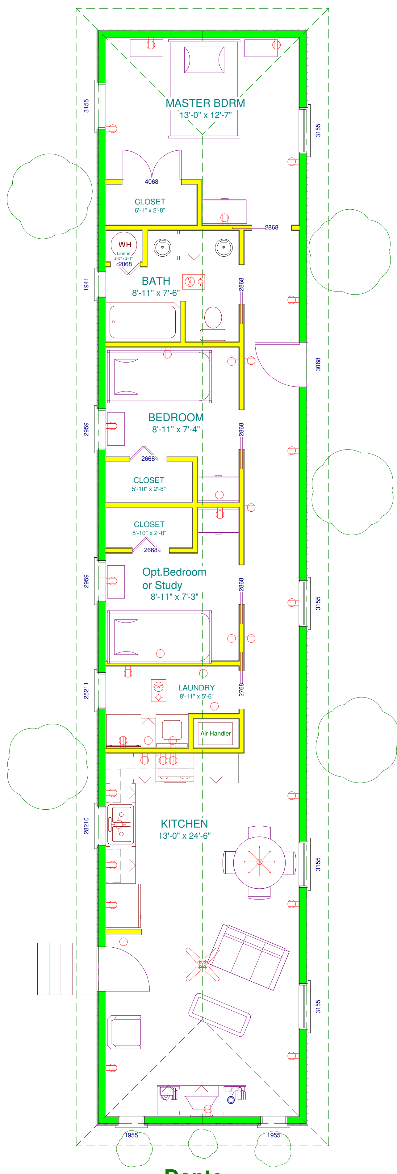
Dante LIVING AREA 1034 sq ft
